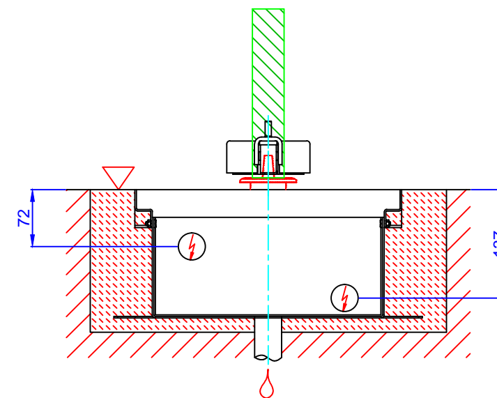
Gecentreerde arm / Bras centrique
