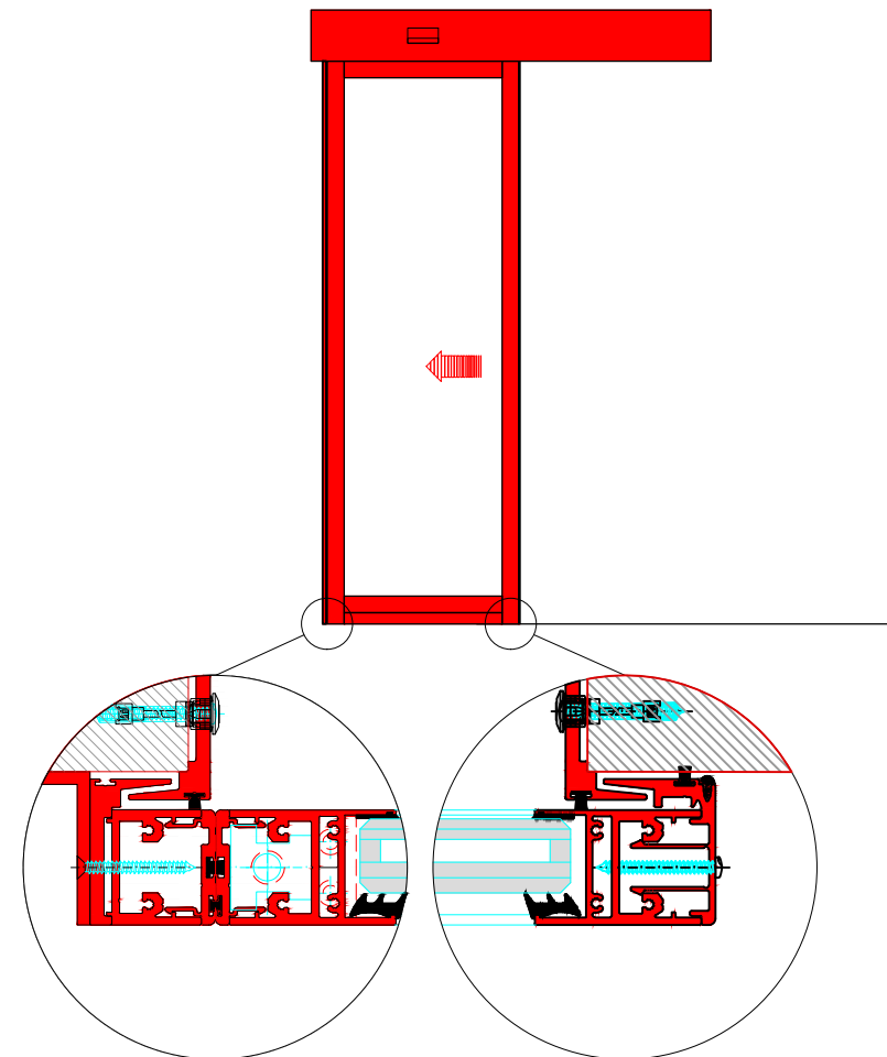
DOORSNEDE A-A / COUPE A-A
