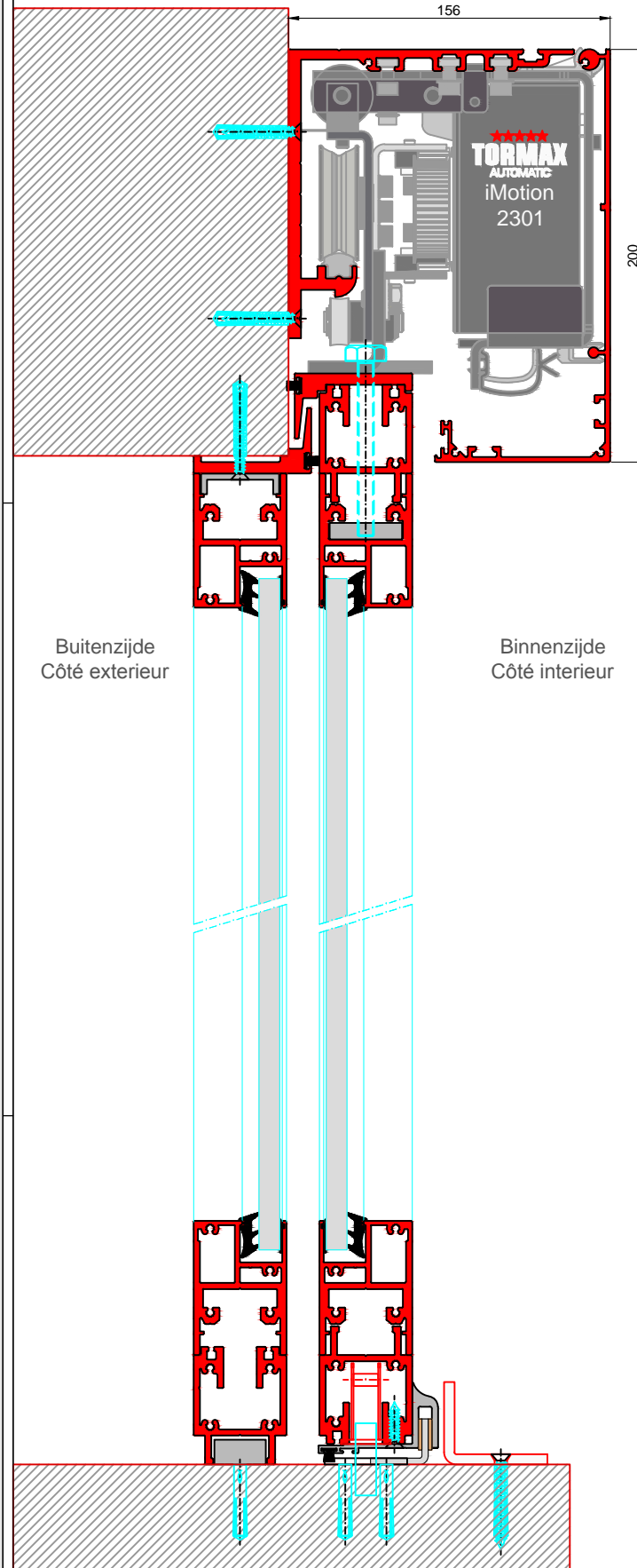
DOORSNEDE B-B / COUPE B-B
