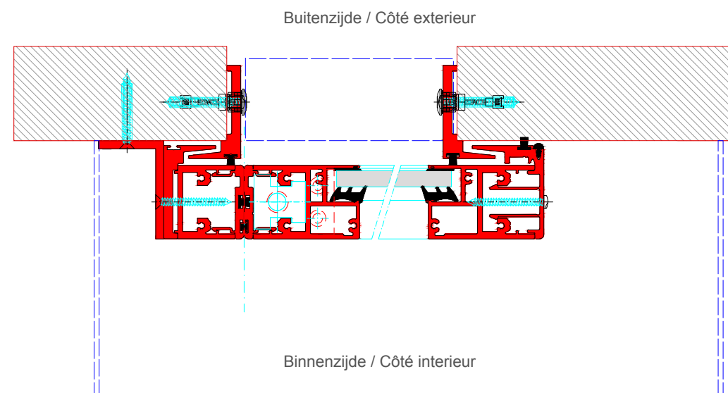
DOORSNEDE A-A / COUPE A-A
