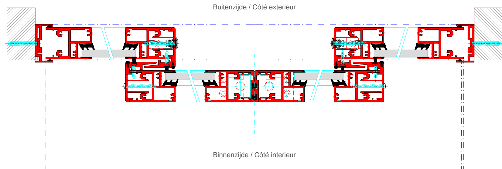
DOORSNEDE A-A / COUPE A-A
