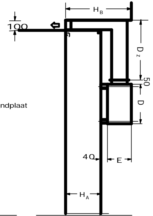
Doorsnede A-A
