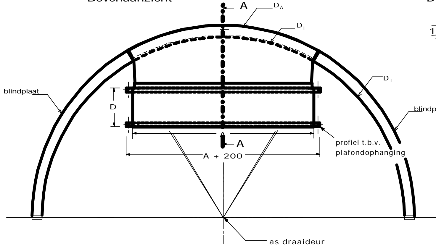
Bovenaanzicht
