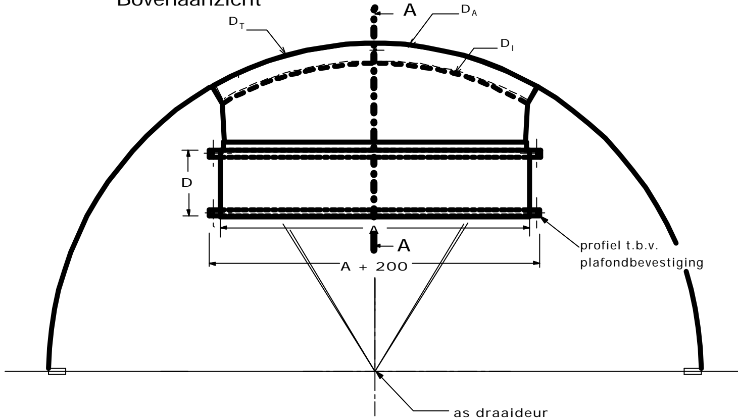
Bovenaanzicht
