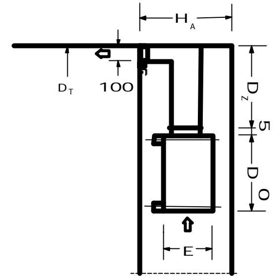
Doorsnede A-A
