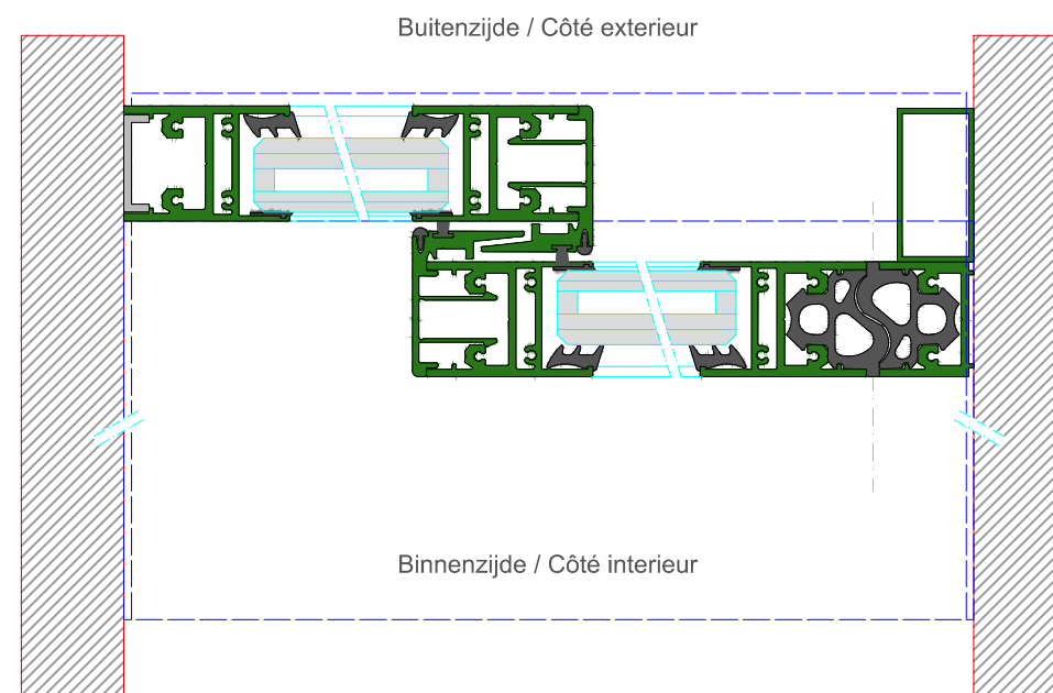
DOORSNEDE A-A / COUPE A-A
