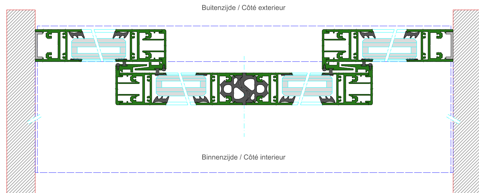
DOORSNEDE A-A / COUPE A-A
