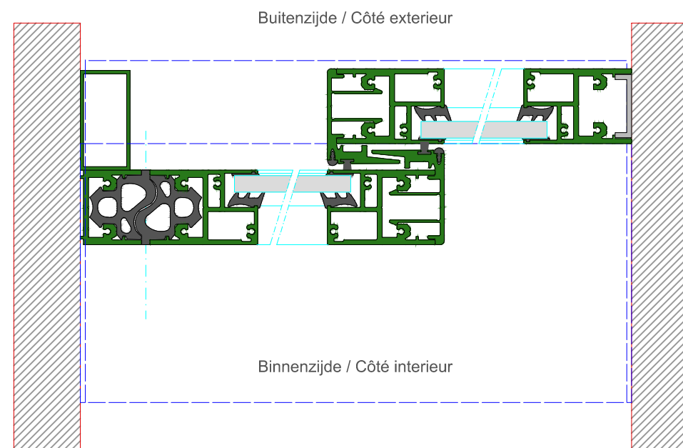
DOORSNEDE A-A / COUPE A-A
