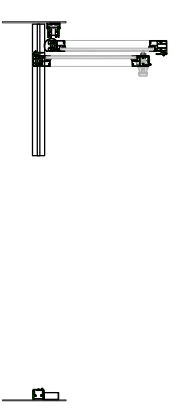
DOORSNEDE A-A / COUPE A-A
