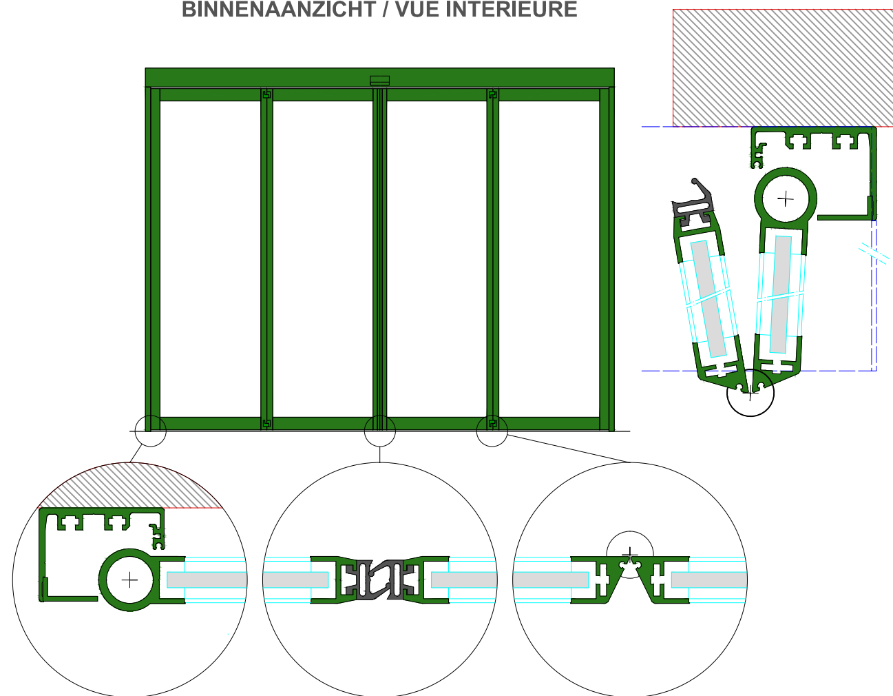
BINNENAANZICHT / VUE INTERIEURE
