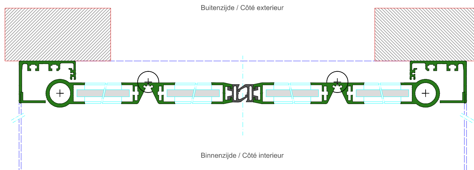
DOORSNEDE A-A / COUPE A-A
