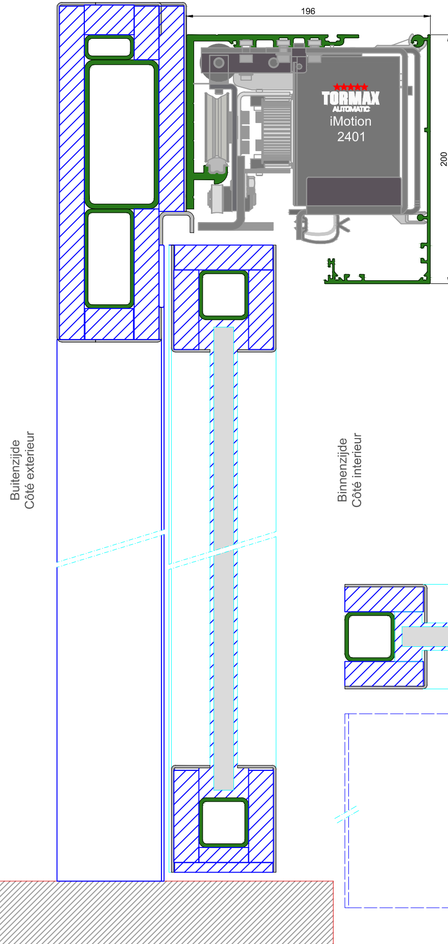
DOORSNEDE B-B / COUPE B-B
