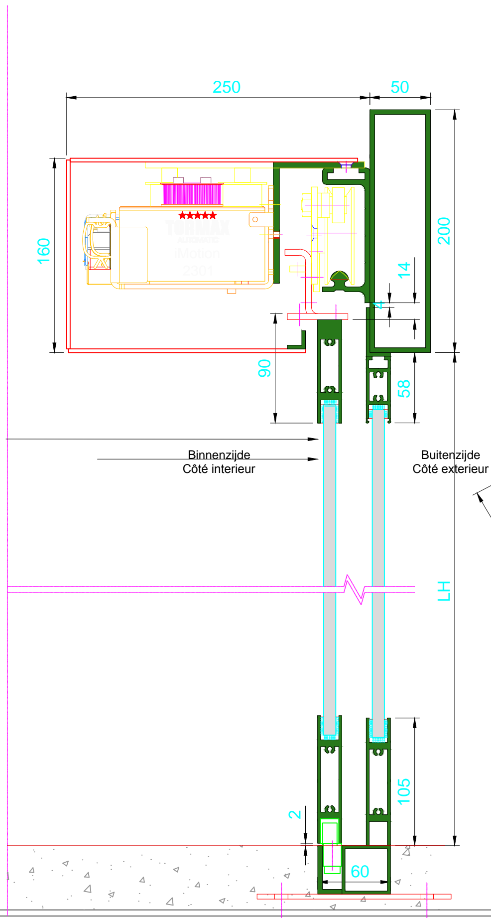
DOORSNEDE D-D / COUPE D-D
