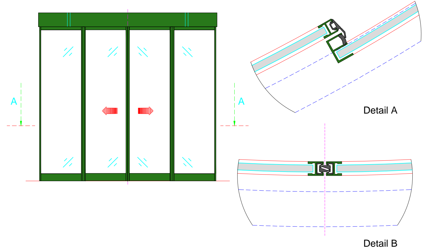
BUITENAANZICHT / VUE EXTERIEURE
