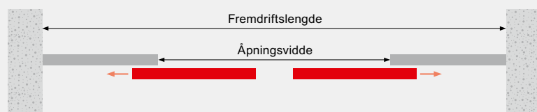
Grunnriss (tofløyet med fast fløyet)
