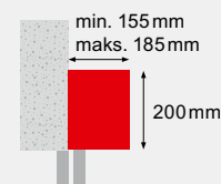
Tverrsnitt
