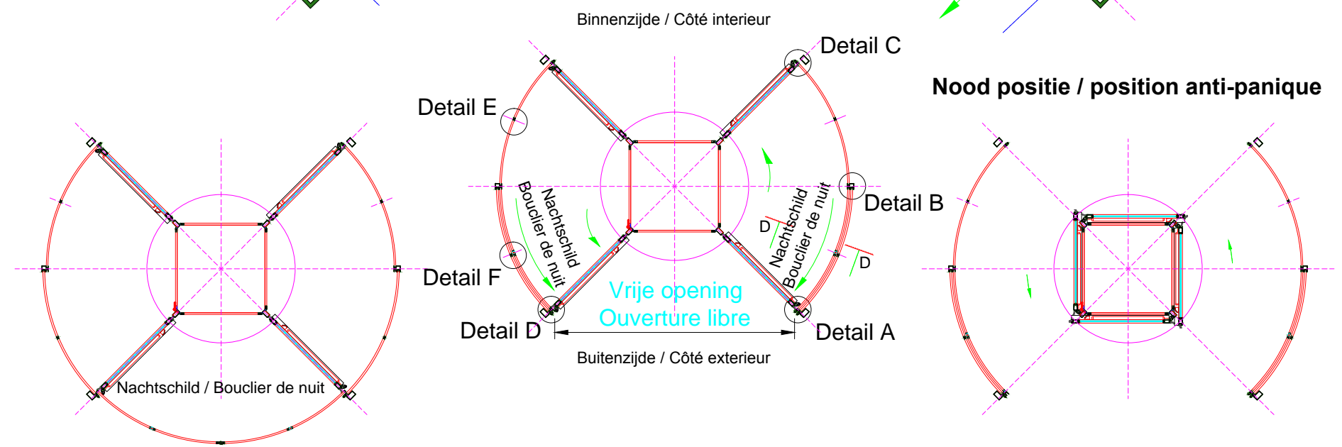
DOORSNEDE A-A / COUPE A-A
